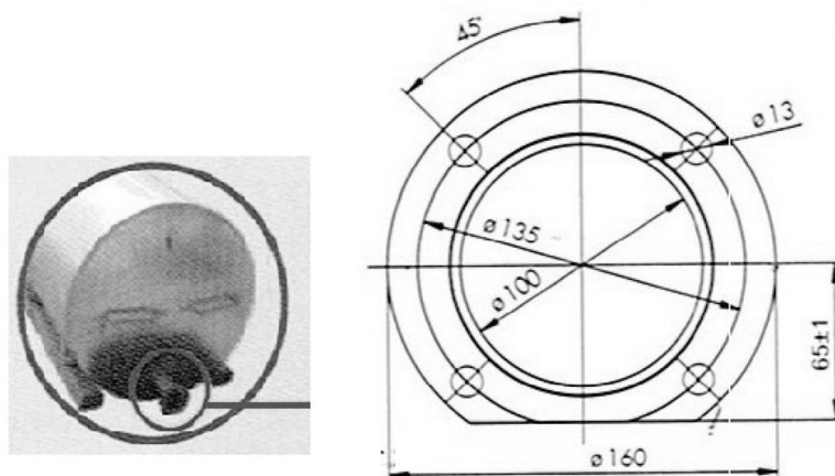
Przekrój zaworu spustowego dla zbiornika 6m 3
